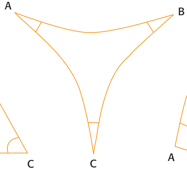
Lobachevsky-Bolyai
