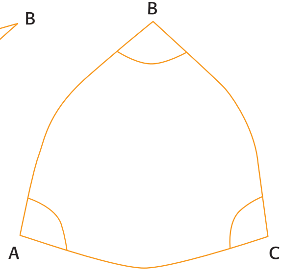
Riemann
