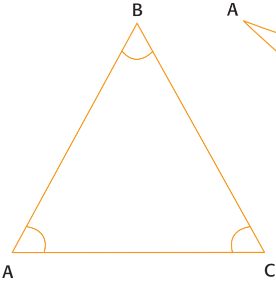
Euclid
